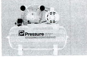
OP 8/50 V-1,5HP Odonto - 1estágio - 120lbs/polP LUBRIFICADO
