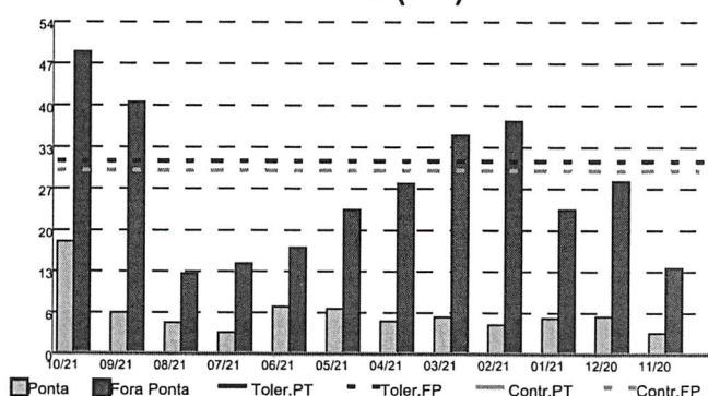
Demanda (kW)
